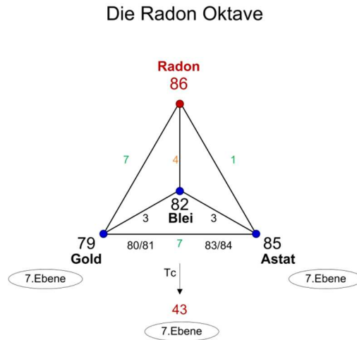
Abbildung 6 Die Tetraederstruktur der Edelgasoktave
