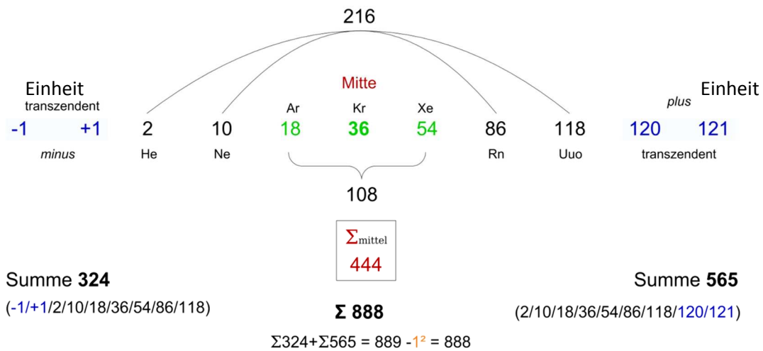
Abbildung 5 die 9 (2 + 7) Edelgase im Periodensystem
